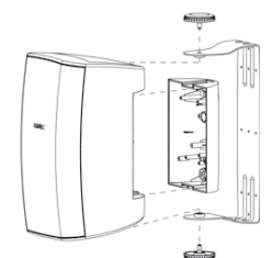
AD-S82 mit U-Bügel /AD-YM8 (T)
