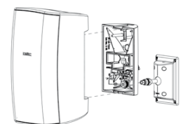
AD-S82 mit Kugelgelenkhalterung
